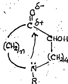
Azaacyloins
